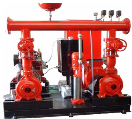
GRUPO BOMBA JOCKEY (2HP) + ELECTRICA (6,5HP) UNE 23-500/90 Hmax: 84Mt - Hmin: 16Mt - Qmax: 22m3/h
